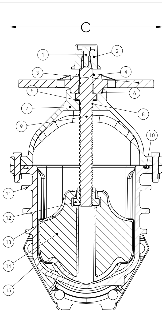
SECTION A-A
